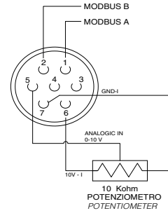
DETTAGLIO CONNESSIONI
